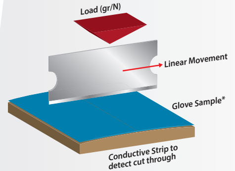
EN388 Coup test
